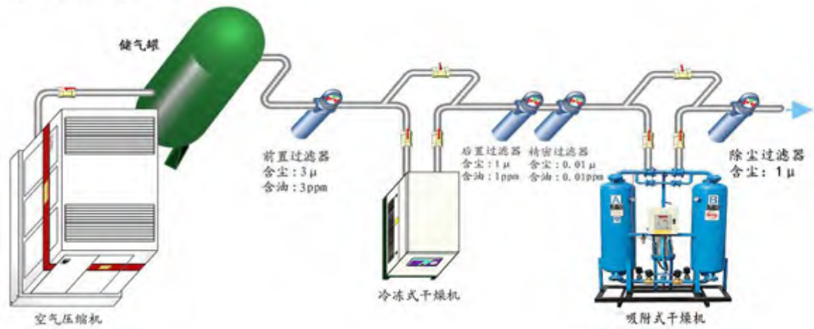
典型高质压缩空气系统图
